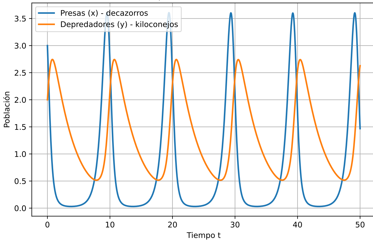
Sistema Depredador-Presa (Lotka-Volterra)
